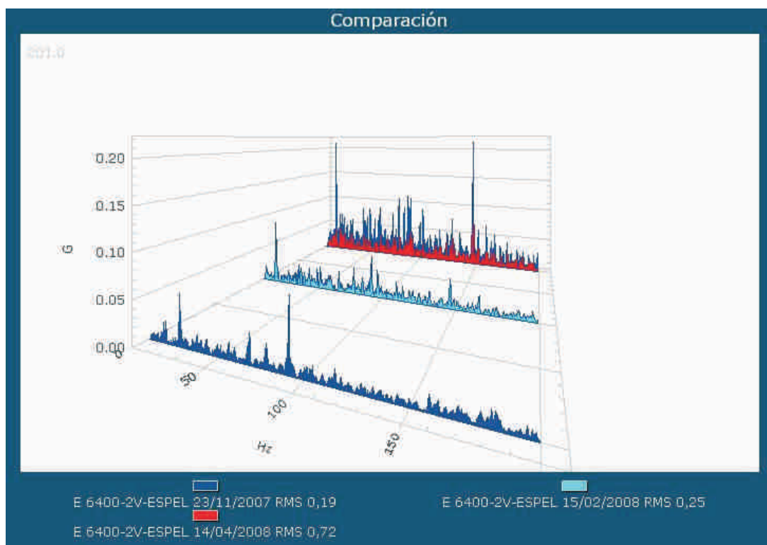
Comparación de los espectros de envoltura tomados en el equipo analizado.
