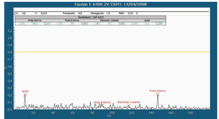
Marcación de las cuatro frecuencias de falla del rodamiento.
