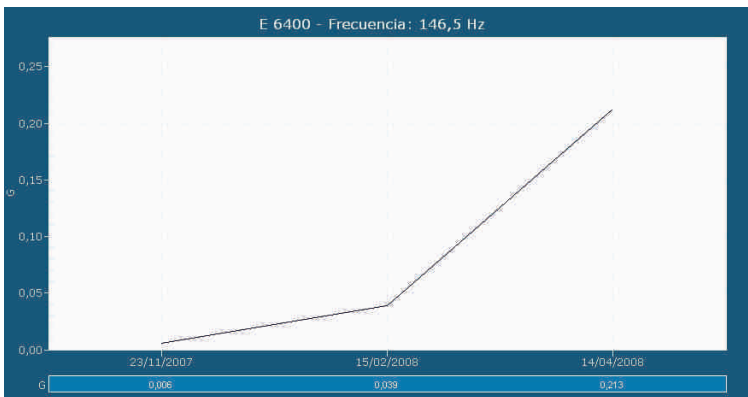
Tendencia del valor de la frecuencia de falla de la pista interna.
